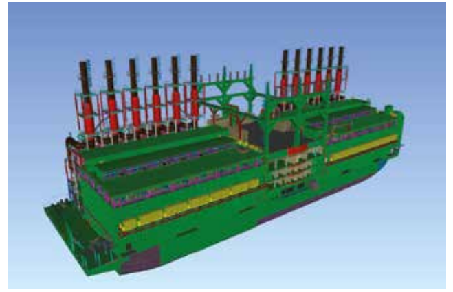
NB23 KARPOWERSHIP 257 MW
